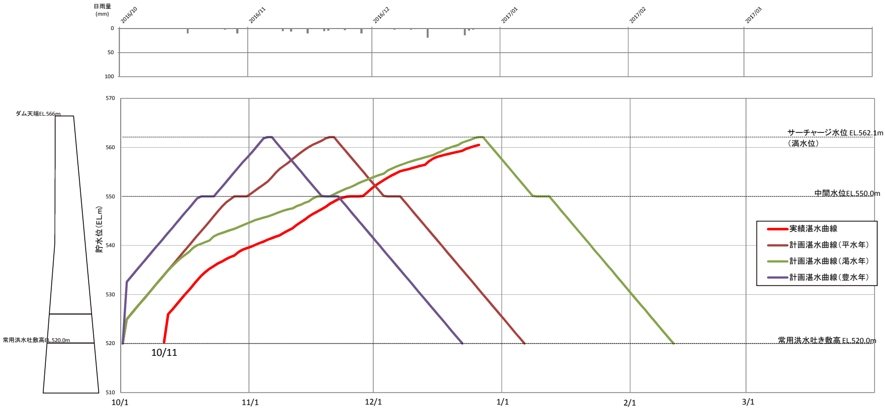
浅川ダム貯留状況図
